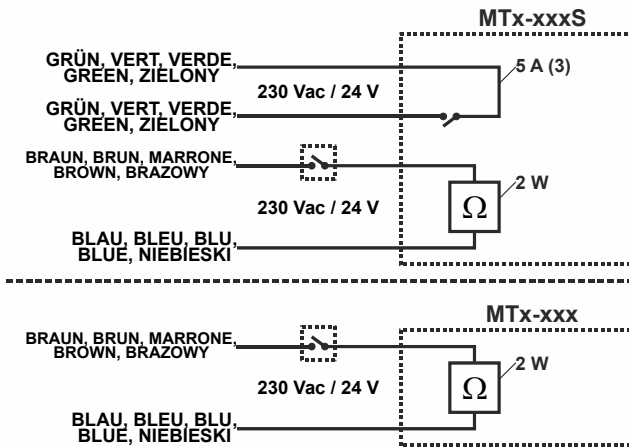
Fig. 4. Wiring diagrams
